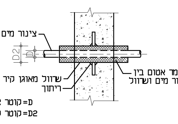
פרם מעבר צינור מים למקלט דרך קיר פנימי
