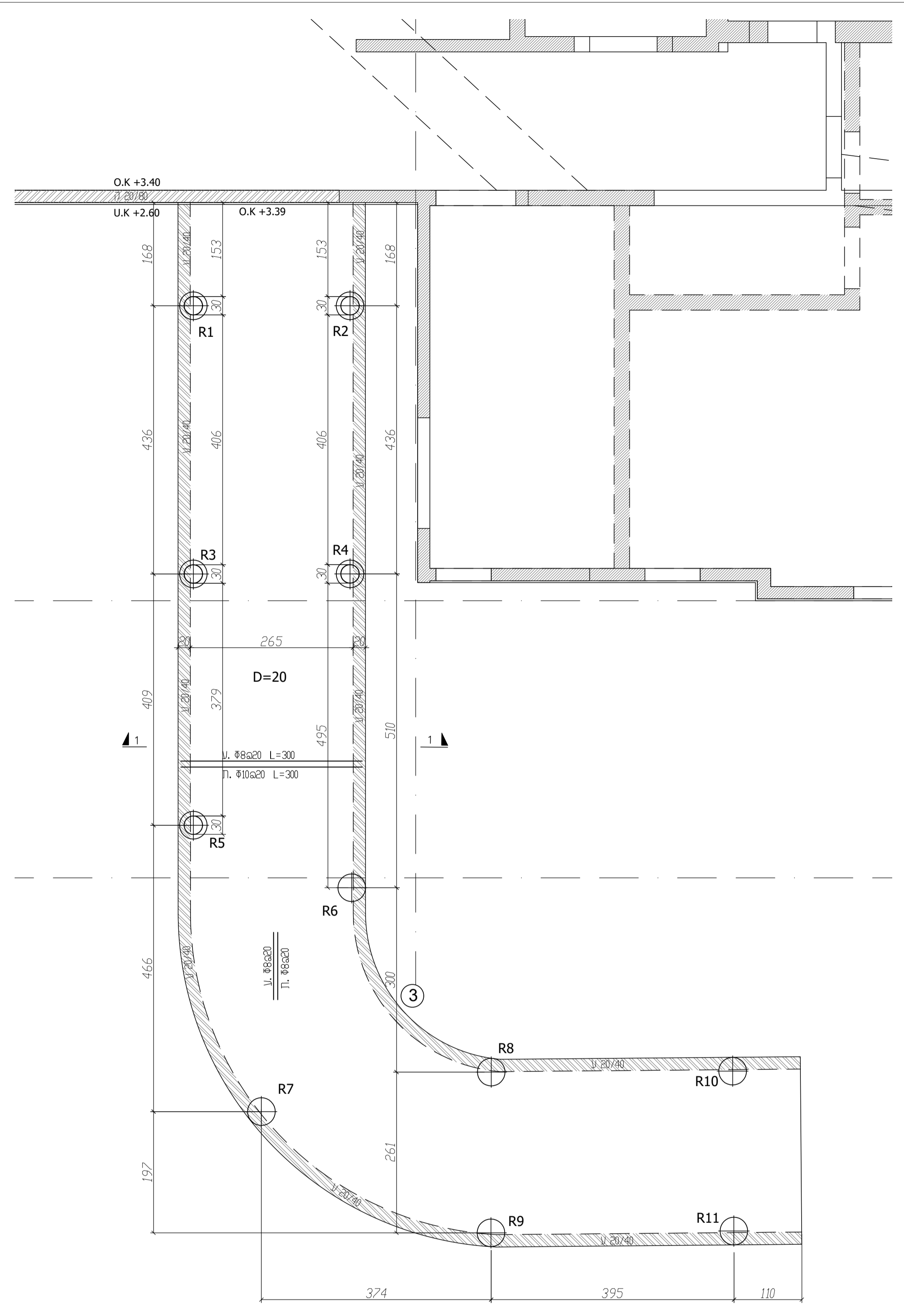
תוכנית רמפה ביצוע מפלסים לפי תוכנית אדריכלית ופיתוח
