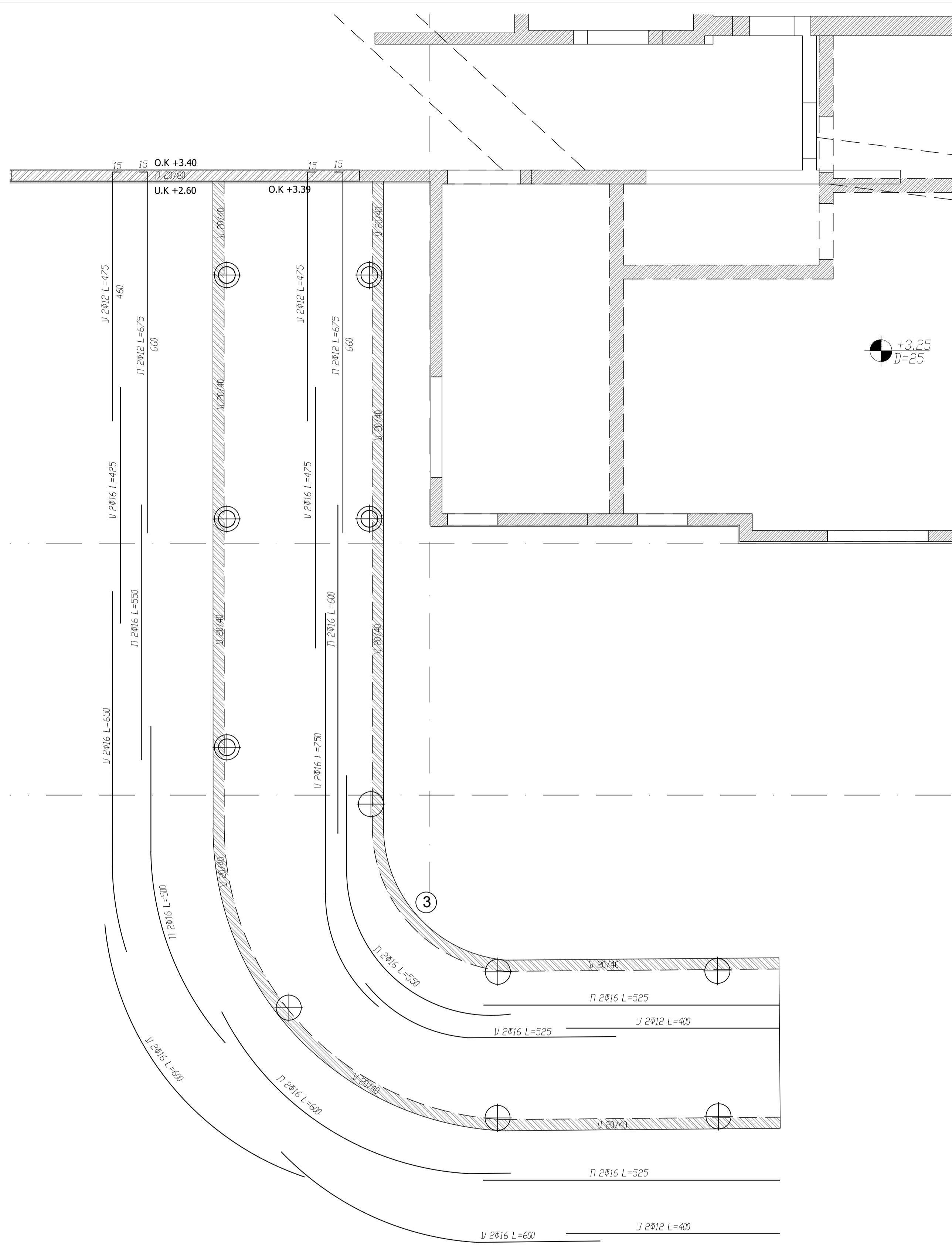
תוכנית זיון קורות
